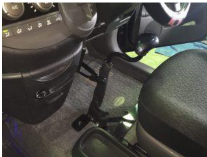
手動式運転装置(下肢損傷)
